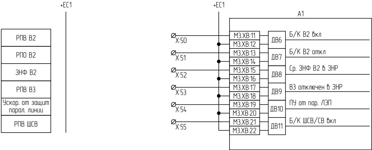
Цепи оперативного тока
