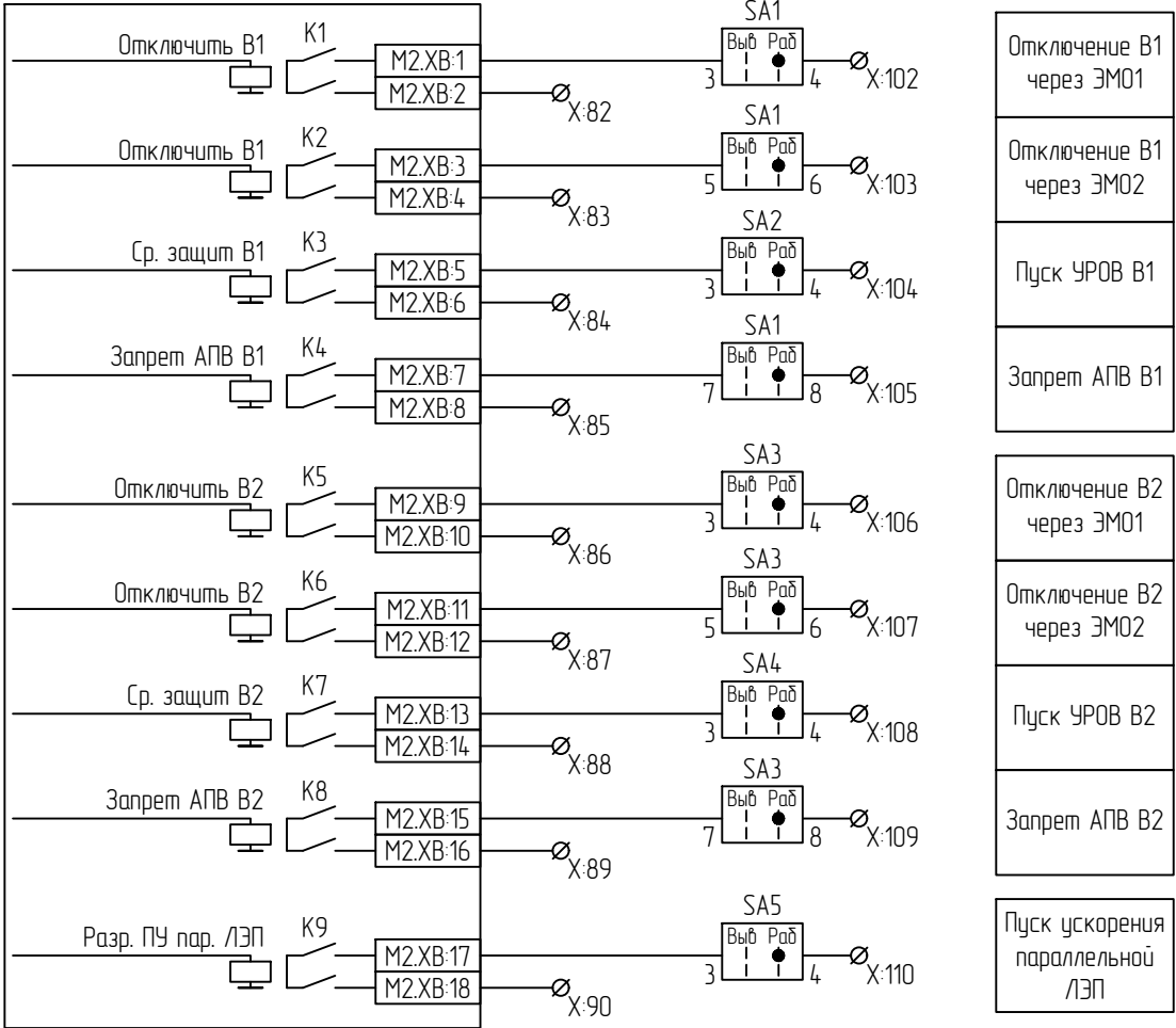
Выходные цепи
